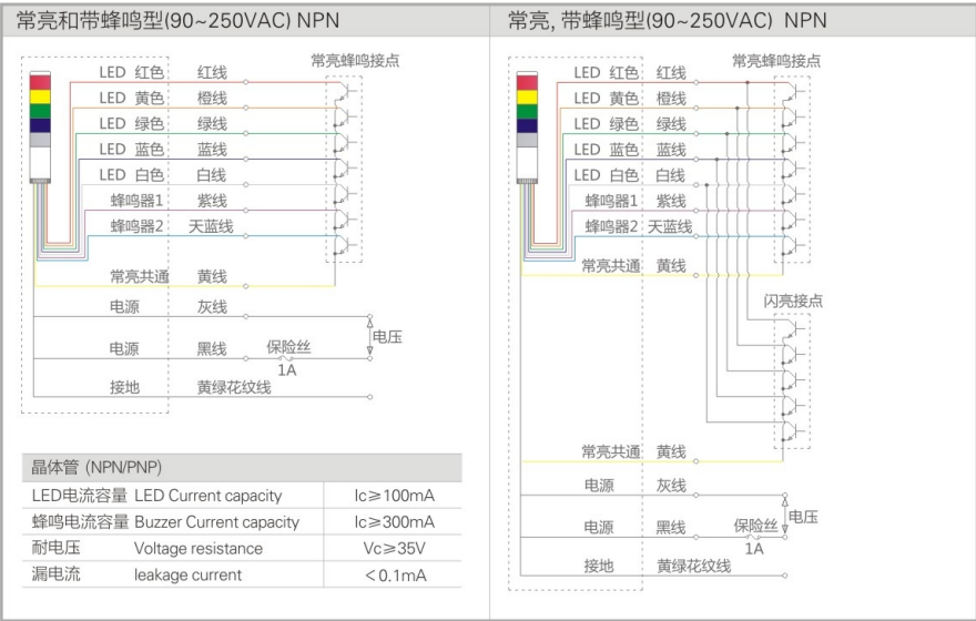
导线颜色对应表 Wire color correspondence table
